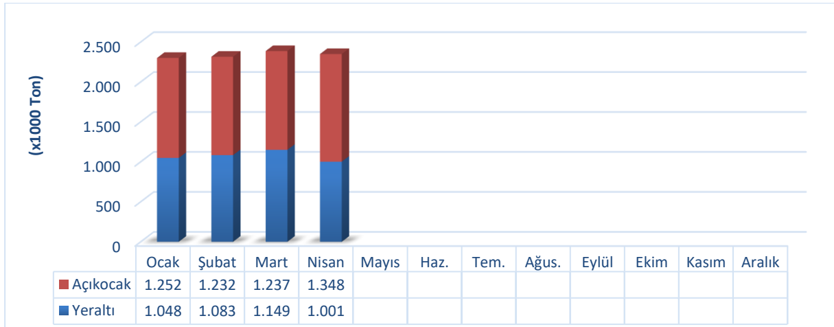
Şekil 4: Aylık Tüvenan Üretim Miktarı (x1000 Ton), 2025
