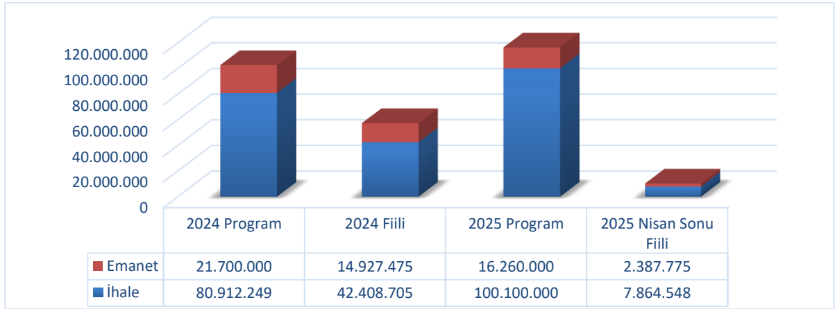
Şekil 1: 2024-2025 Karşılaştırmalı Dekapaj Miktarları (m 3 )
