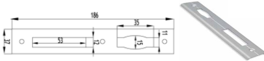
C60 Makaralı Kilit Karşılığı Teknik ve Temsili Resim
